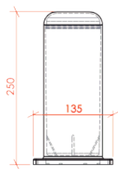
BOLARDO BAJO 3,45 Kg
