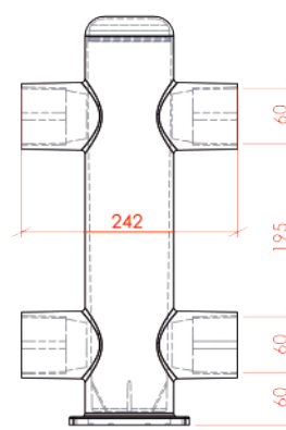
BOLARDO ALTO 4 SALIDAS 5,89 Kg
