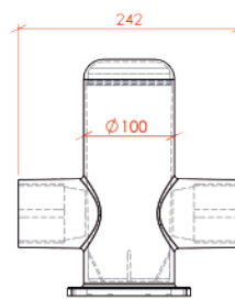
BOLARDO BAJO 2 SALIDAS 3,65 Kg
