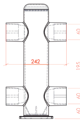
BOLARDO ALTO 4 SALIDAS 3,00 Kg
