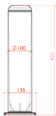
BOLARDO ALTO 2,60 Kg
