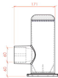
BOLARDO BAJO 1 SALIDA 1,45 Kg
